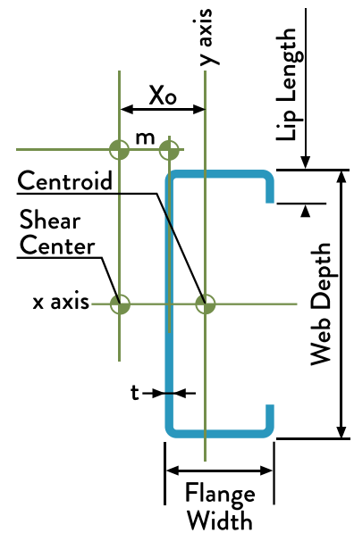
Stud Cross Section
